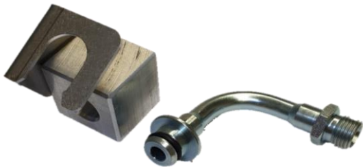
Adapter 400.470.000 Anschluss zwischen Ölkühlerleitung und Getriebe Connection between oil cooler line and transmission
