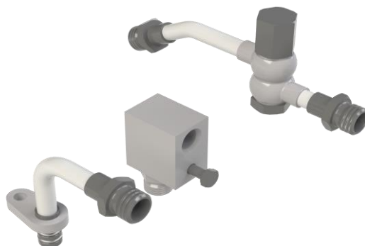
Adapter 400.433.000 *** Anschluss zwischen Ölkühlerleitung und Getriebe Connection between oil cooler line and transmission
