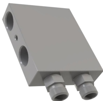
Adapter 400.498.000 Anschluss anstelle des Thermostats Connection instead of the thermostat
