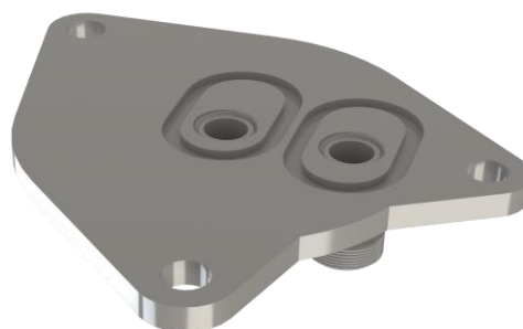
Adapter 400.477.000 Anschluss anstelle des Ölkühlers Connection instead of oil cooler
