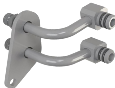
Adapter 400.469.000 Anschluss anstelle des Ölkühlers
